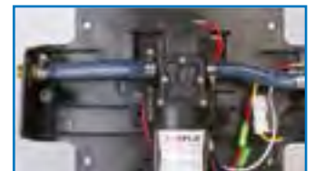
Bomba de membranas
